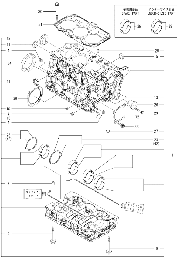
OCD50-M00330 3TNM74F-SAFS Fig.1. CYLINDER BLOCK
