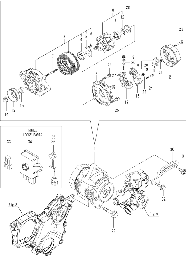
Fig.15. GENERATOR
